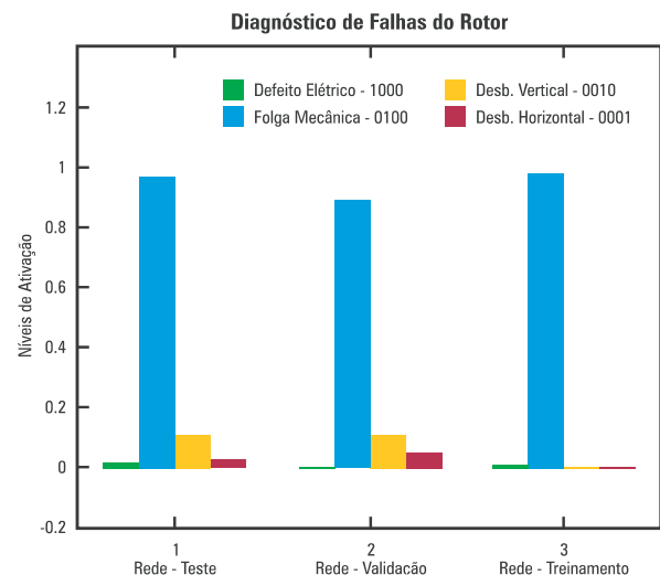
Figura 4. Folga Mecânica
