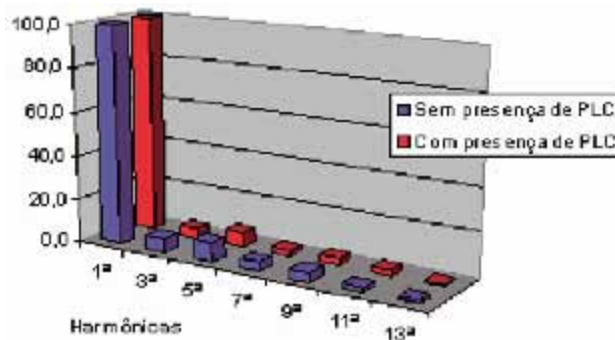
Figura 9. Diagrama espectral das harmônicas presentes na corrente da terceira fase até a 13ª harmônica
