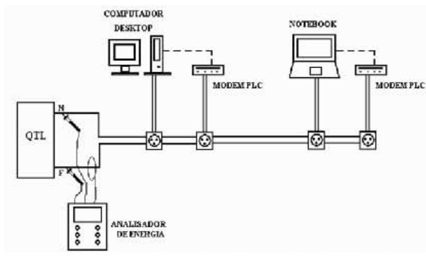
Figura 2. Diagrama para medição no QTL
