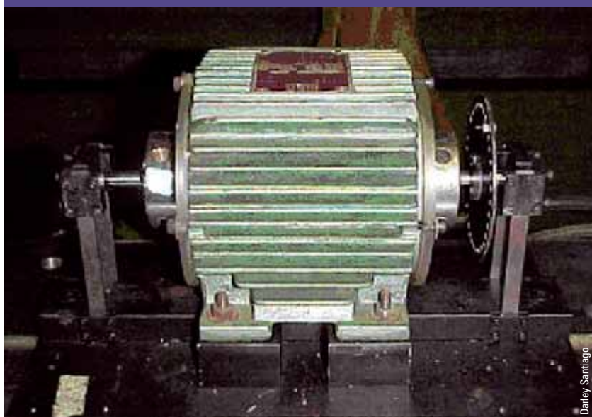
Figura 1. Bancada experimental de testes
