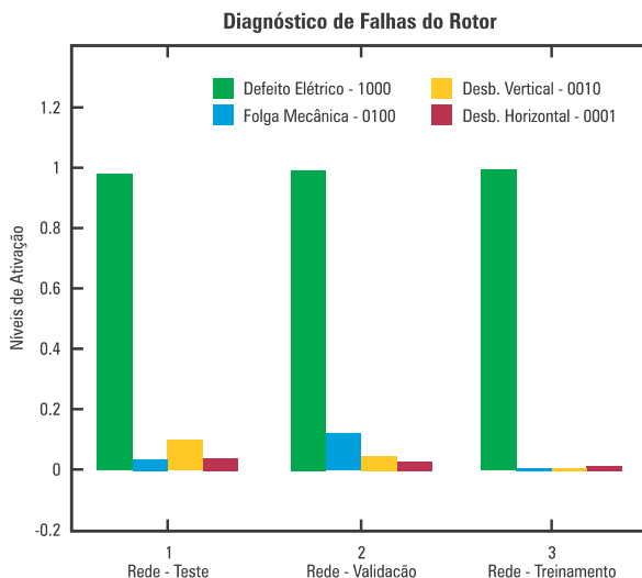
Figura 3. Defeito Elétrico
