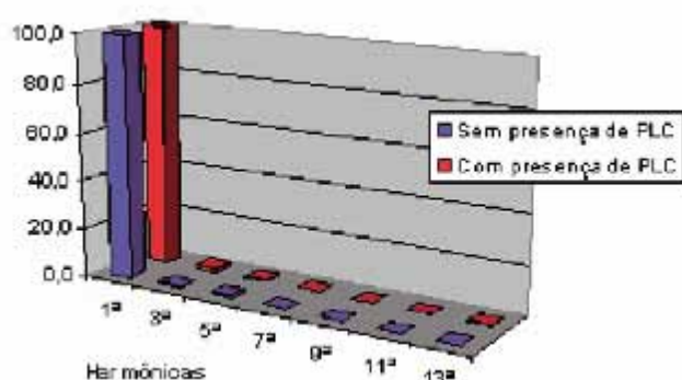
Figura 4. Diagrama espectral das harmônicas presentes na tensão da primeira fase até a 13ª harmônica
