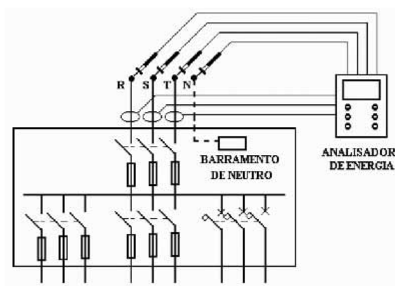
Figura 3. Diagrama para medição em um quadro trifásico
