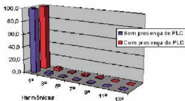
Figura 7. Diagrama espectral das harmônicas presentes na corrente da segunda fase até a 13ª harmônica
