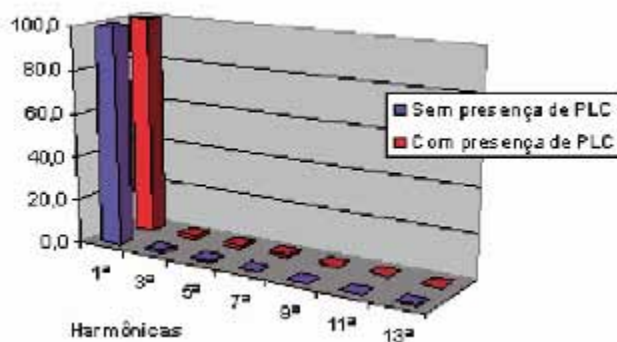
Figura 6. Diagrama espectral das harmônicas presentes na tensão da segunda fase até a 13ª harmônica
