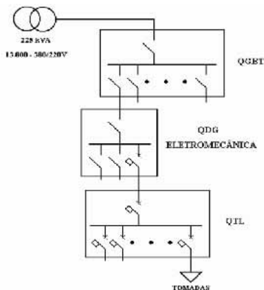
Figura 1. Diagrama unifilar das instalações elétricas envolvidas nas medições
