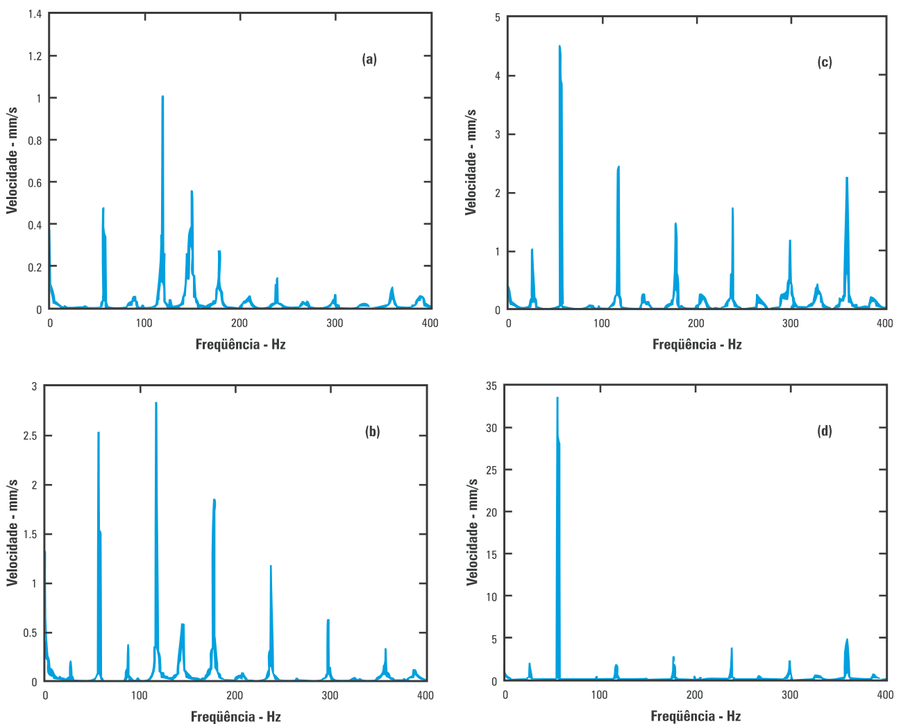
Figura 2. Espectros do Defeito Elétrico (a); Folga Mecânica (b); Desbalanceamento Vertical + Folga Mecânica (c) e Desbalanceamento Horizontal (d)
