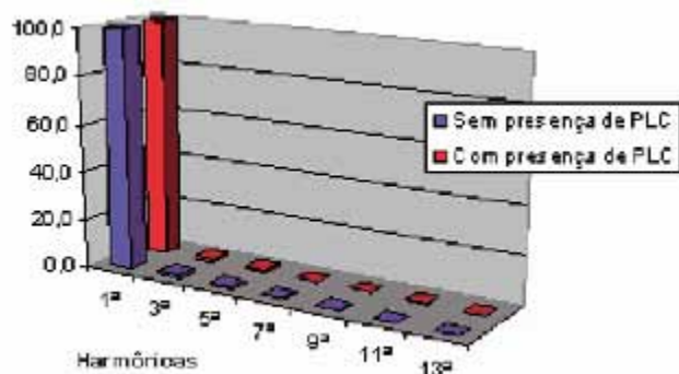
Figura 8. Diagrama espectral das harmônicas presentes na tensão da terceira fase até a 13ª harmônica
