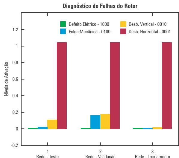
Figura 6. Desbalanceamento Horizontal
