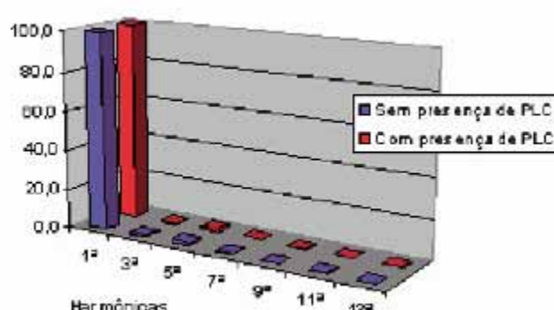
Figura 5. Diagrama espectral das harmônicas presentes na corrente da primeira fase até a 13ª harmônica
