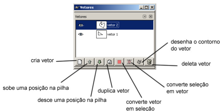
Figura 135 - janela com caixa de diálogo “vetores”.
