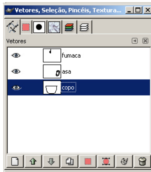
Figura 166 - vetor "copo" selecionado na camada referente à caixa de diálogos de "vetores". O ícone quadrado em vermelho cria uma seleção a partir do vetor. Os ícones de olhos significam que os vetores estão visíveis na janela de imagem
