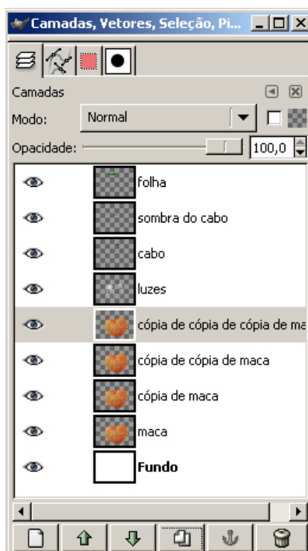
Figura 59 - camadas duplicadas assumem os nomes de “cópia de” + nome da camada que deu origem à duplicação.
