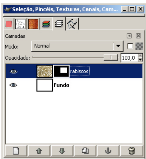
Figura 84 - camada "rabisco" com janela da máscara. Note que a camada permanece com toda a informação sobre o que está oculto pela máscara.
