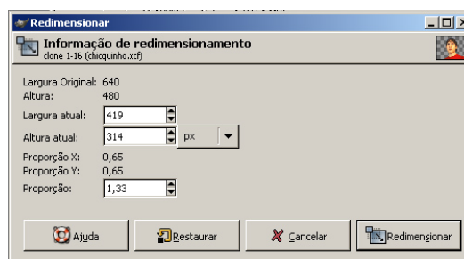
Figura 197 - caixa de diálogo que aparece quando usamos a ferramenta redimensionar. Essa caixa permite que o redimensionamento seja feito com precisão através da configuração de valores específicos.
